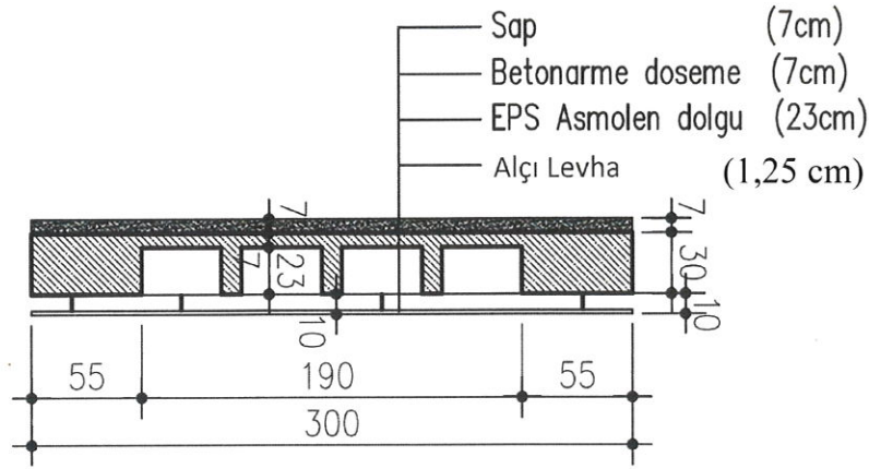
Şekil-4 Alçı panelli sistem enine kesit
